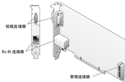
图 1-2. DRAC 4/P 硬件配置
