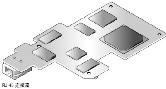
图 1-2. DRAC 4/P 硬件配置
